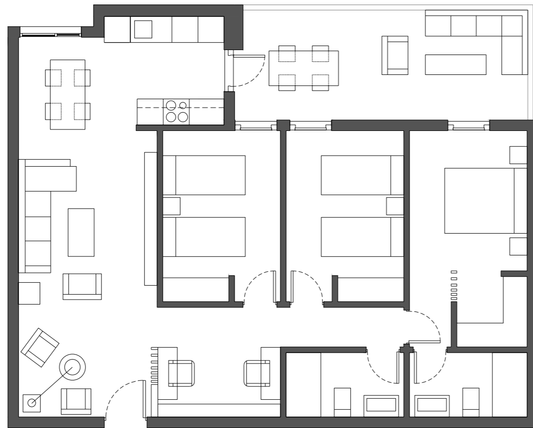
Planta Distribución
