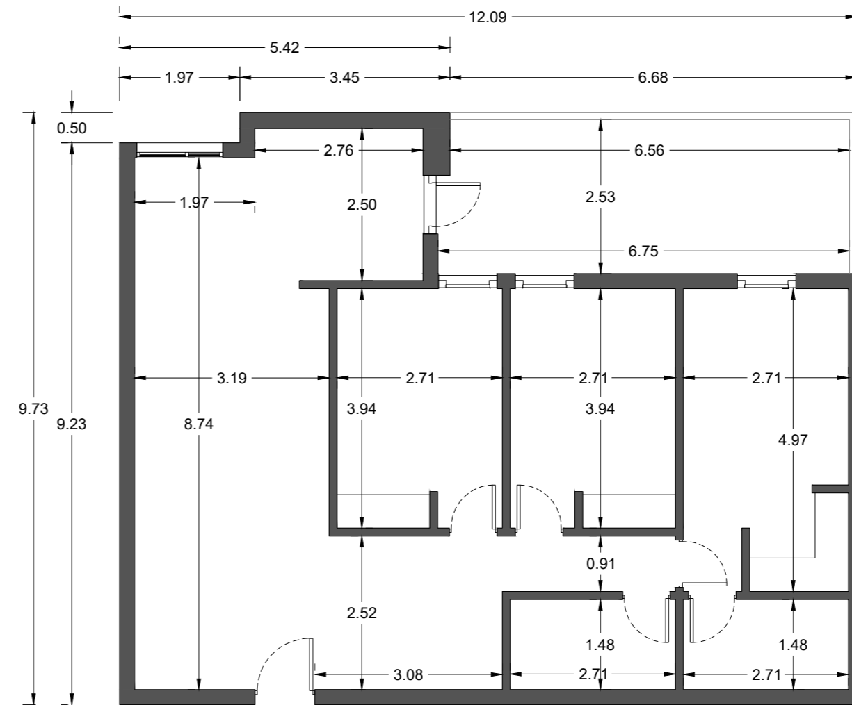
Planta Cotas
