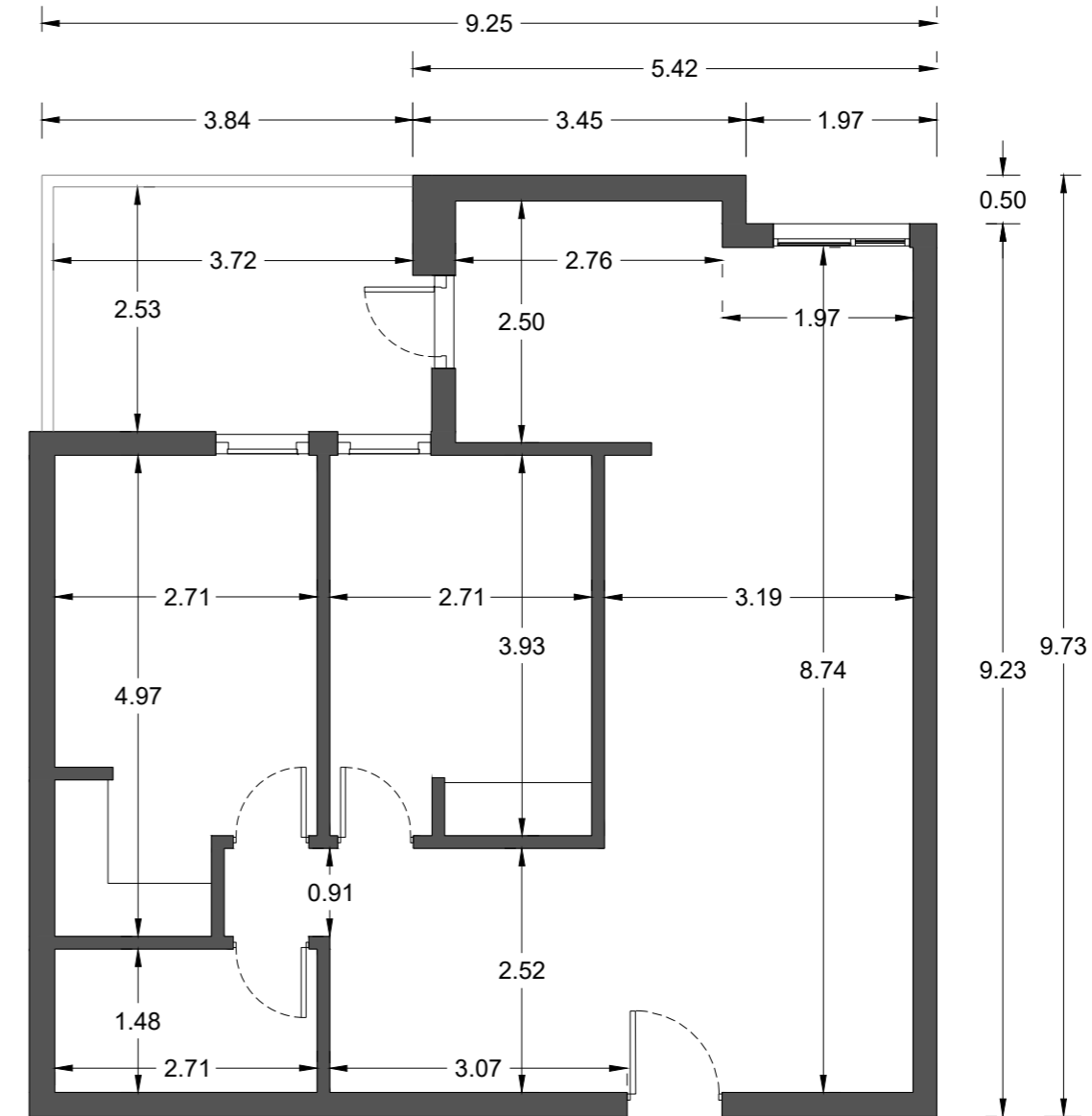
Planta Cotas
